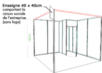
Stand type de 9m 2 avec réserve de 1m 2
